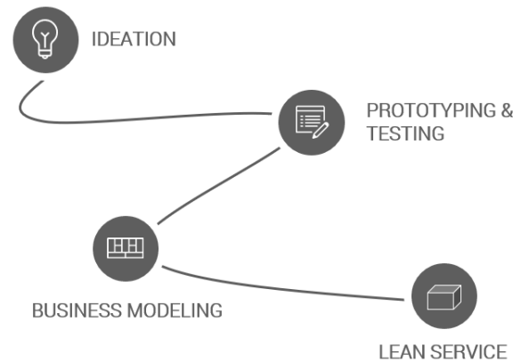
Abbildung 1: Lean-Service-Creation-Ansatz
